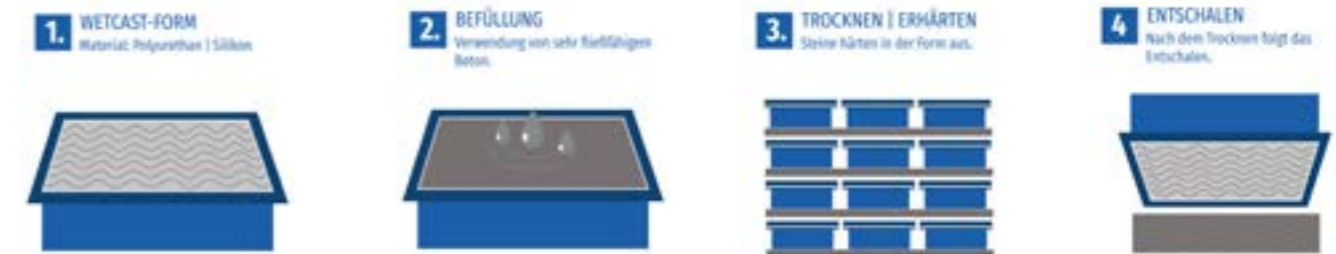
Abbildung 3: 1. Verwendung spezieller Wetcast-Formen | 2. Befüllung mit sehr fließfähigem Beton | 3. Erhärten und Trocknen in der Form | 4. Entschalen und Wiederverwenden der Form
